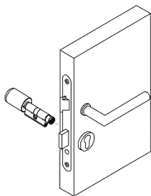
Abbildung 1: Den Zylinder einsetzen
