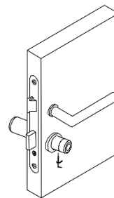
Abbildung 3: Den Knauf befestigen
