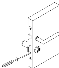
Abbildung 2: Den Zylinder fixieren
